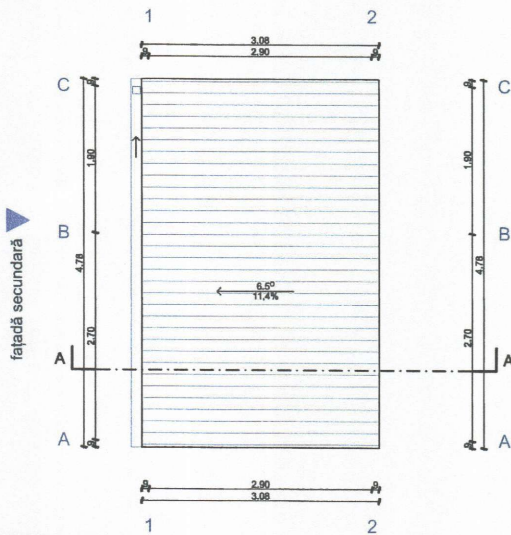
PLAN ÎNVELITOARE, SC.1:50
